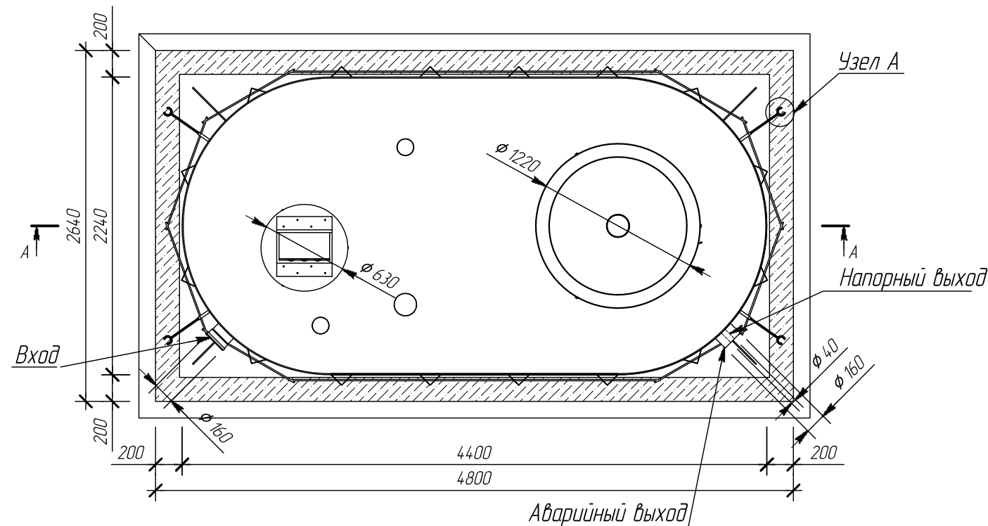
Вид сверху
