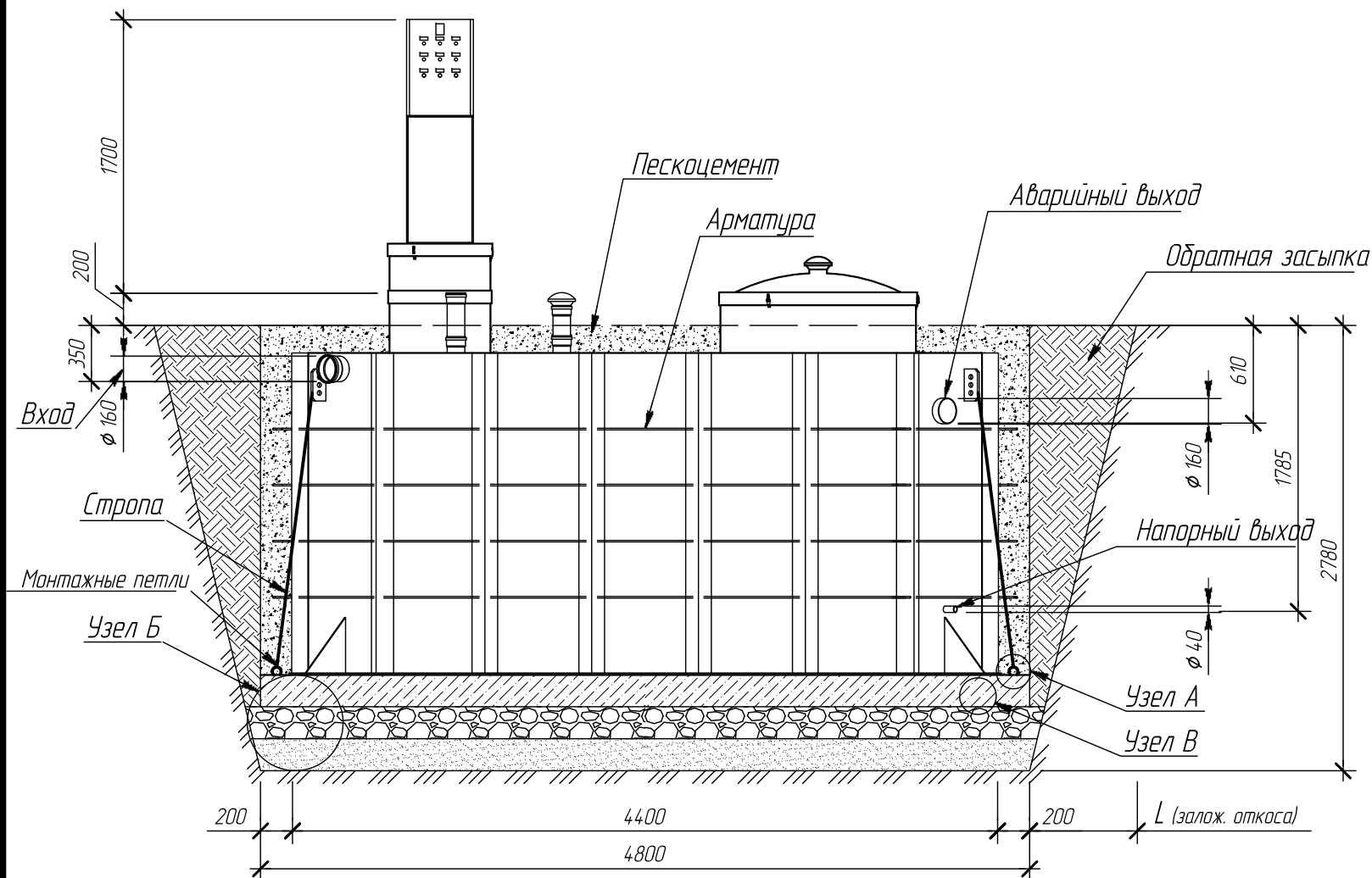
Разрез А-А по котловану
